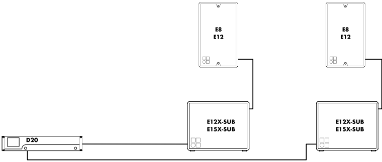
D20 amplifier in Mix TOP/SUB mode with E8 or E12 loudspeakers and E12X or E15X subwoofers
